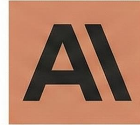
Claude
